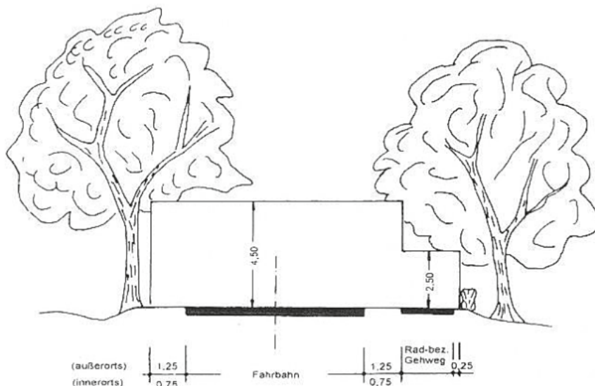
Lichtraumprofil
