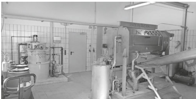
Neue Schneckenpresse mit neuer Polymeransatzstation (Linke Bildhälfte) und Steuerungsschrank im Hintergrund
